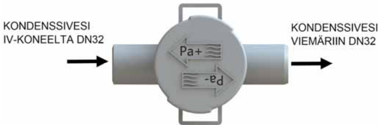
Kuva 17. Pingispallovesilukon asennussuunta
