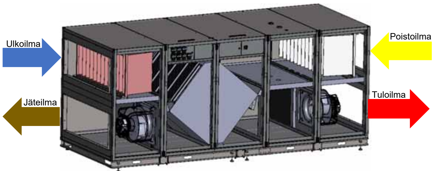
Kuvassa pyöreä tulo ja pyöreät lähdöt. Lähtöjärjestys -L
