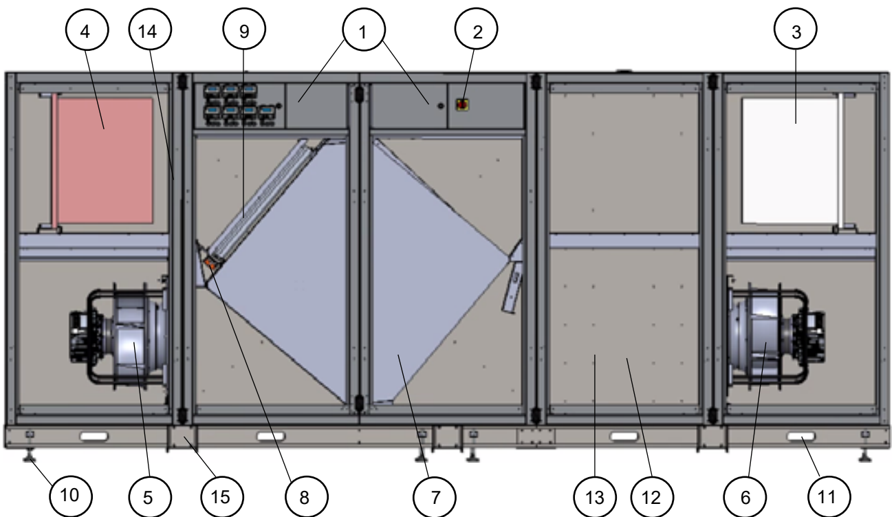
Kuva 21. Vasenkätinen IV-kone.
