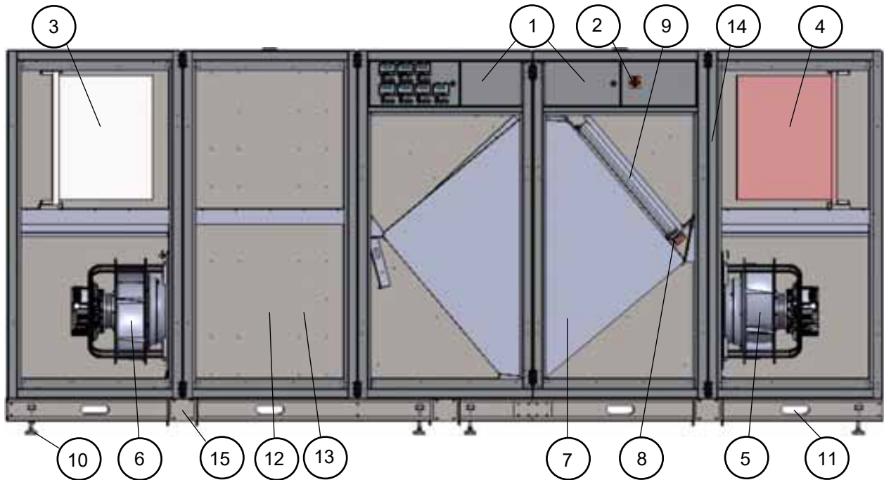
Kuva 20. Oikeakätinen IV-kone.
