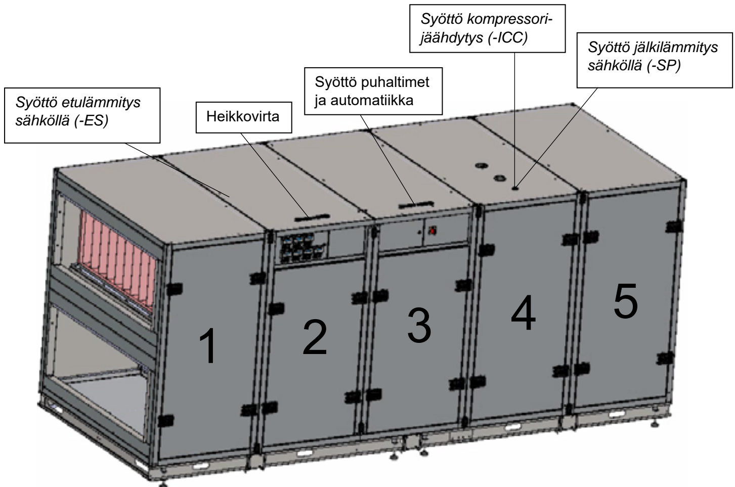
Kuva 9. Sähkösyötöt Kuvassa esimerkkinä vasenkätinen (-L) IV-kone kanttilähdöillä.
