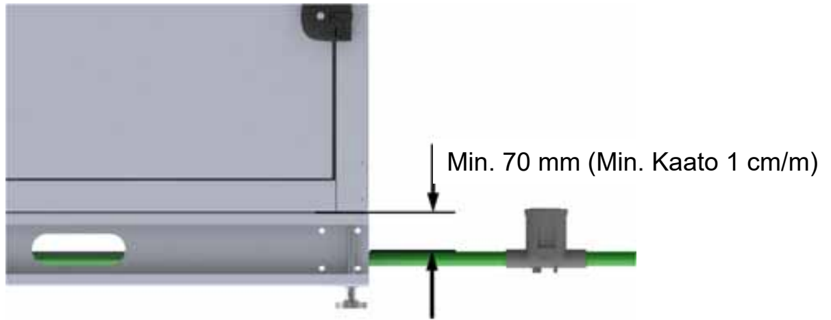
Kuva 15. Kondenssivesiputken kaato
