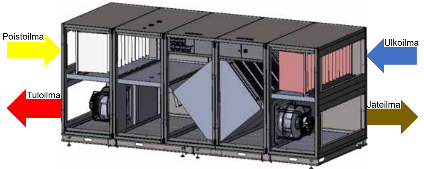
Kuvassa kantitulo ja kantilähdöt. Lähtöjärjestys -R
