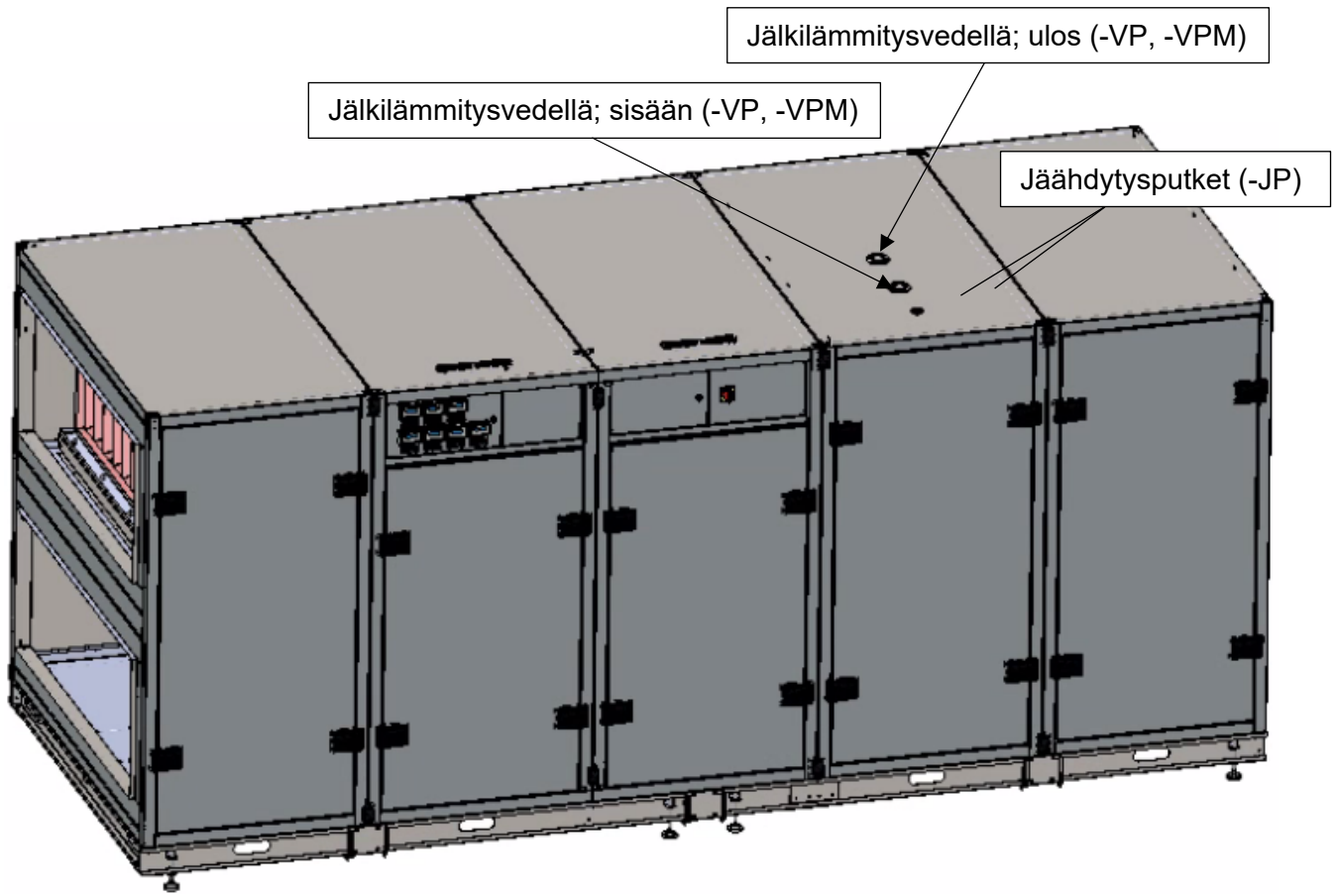
Kuva 18. Vesipatterijäähdytyksen läpiviennit. Kuvassa esimerkkinä vasenkätinen IV -kone.
