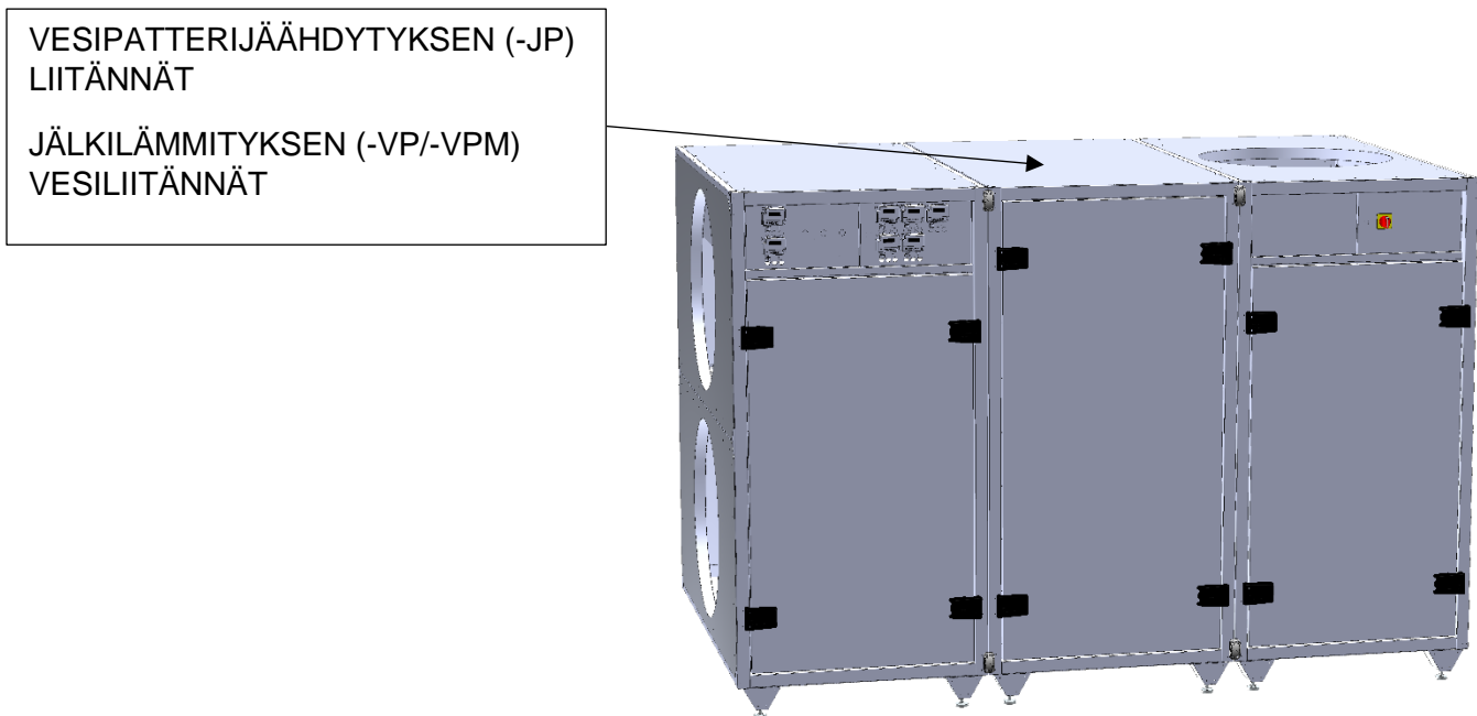
Kuva 5.8 Jälkilämmityksen ja vesipatterijäähdytyksen liitännät. Kuvassa esimerkkinä lähtöjärjestys R.
