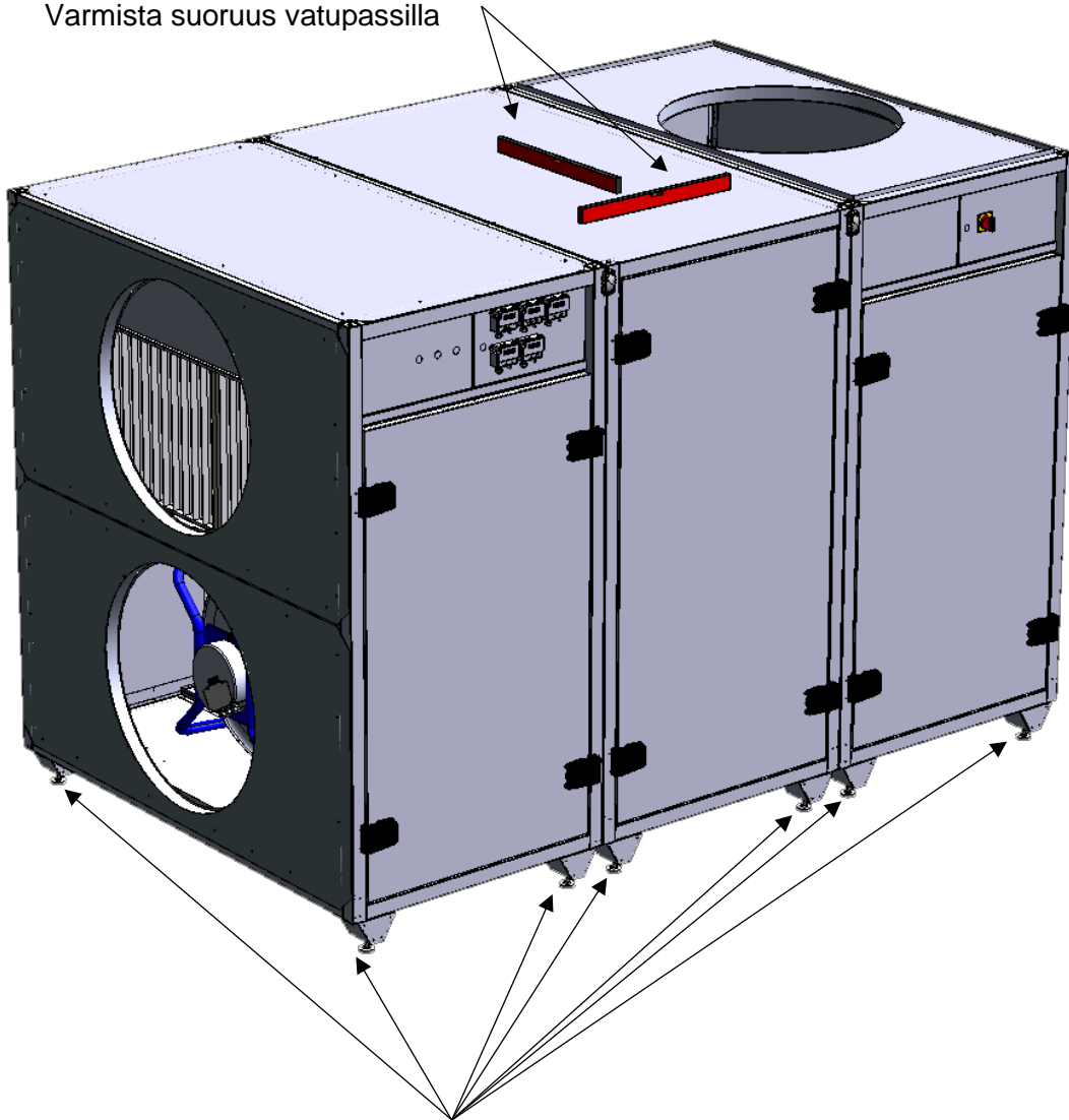
Kuva 5.2 Koneen vaakasuoruus varmistetaan vatupassilla
