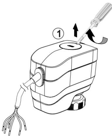
Kuva 7.3 Toimilaite
