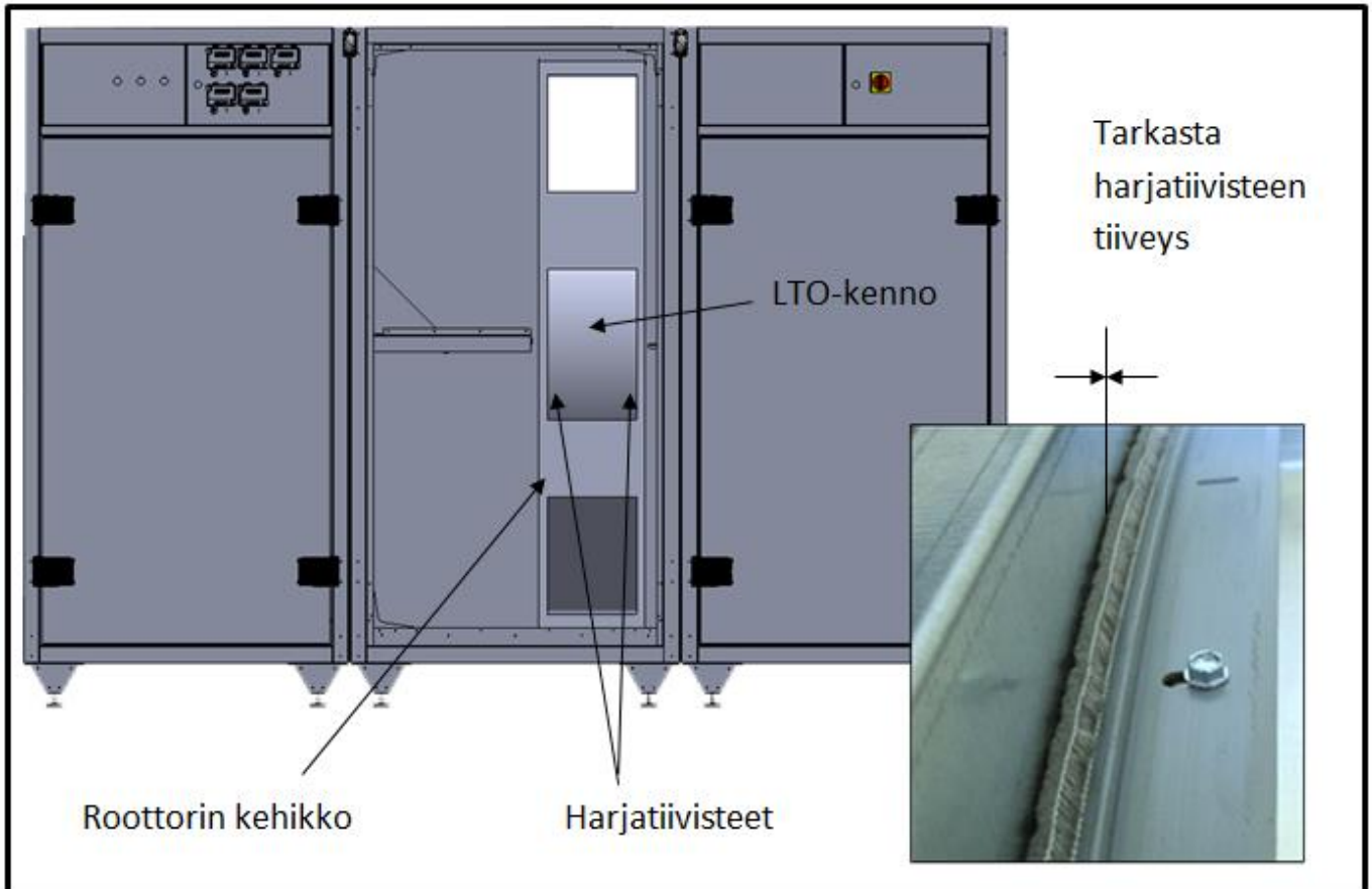
Kuva 7.1 LTO-roottori
